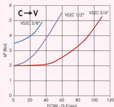
PERDITE DI CARICO PRESSURE DROPS CURVE
